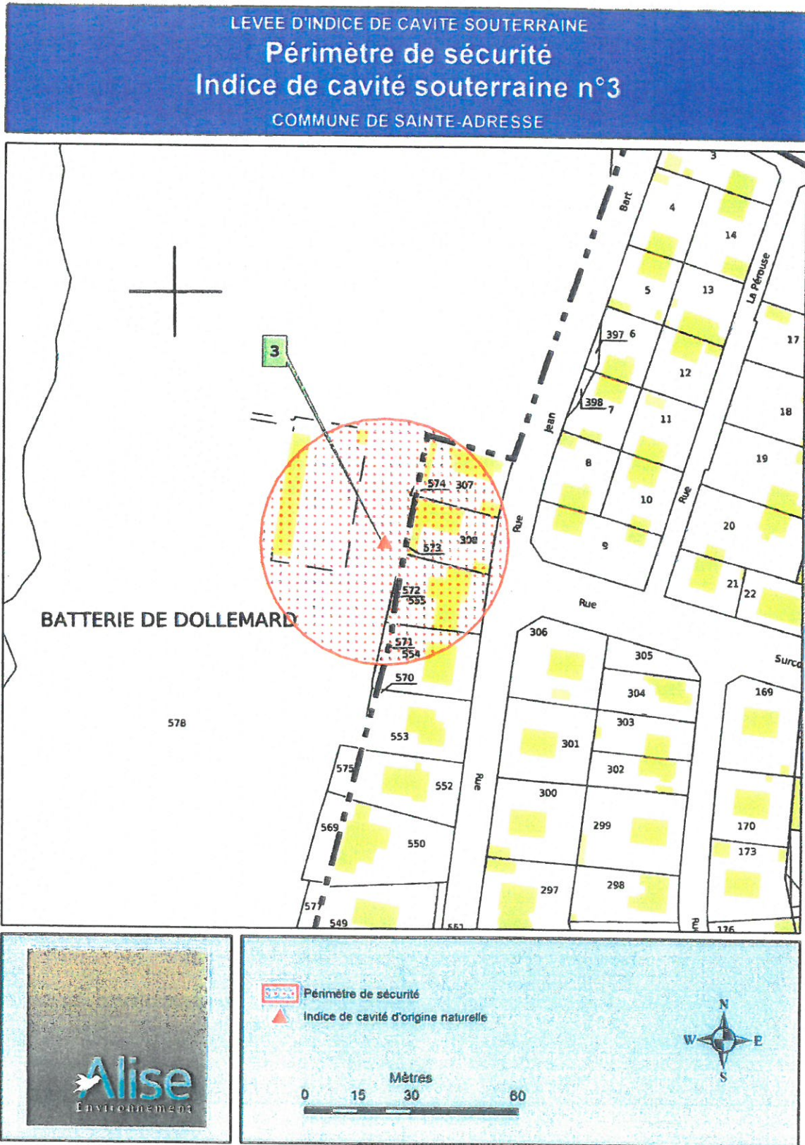
Figure 3 : Périmètre de sécurité avant travaux de décapage
